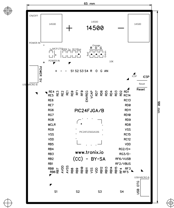
PIC24FJGA/B - (02/2018) - SCALE: 100%
