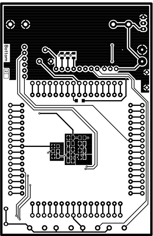
PIC24F1020B - (05\5018) - SCALE: 100%
