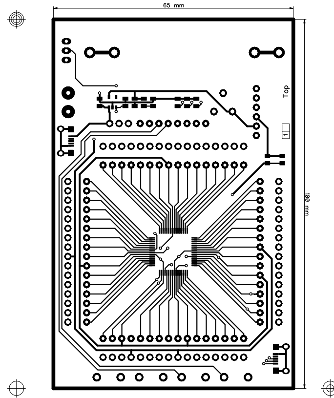
PIC24FJGA/B - (02/2018) - SCALE: 100%
