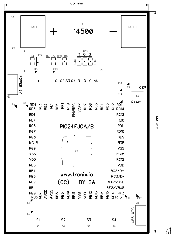
PIC24FJGA/B - (02/2018) - SCALE: 100%
