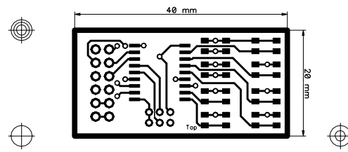
MCP23S08-SWITCH - (09/2017) - SCALE: 100%
