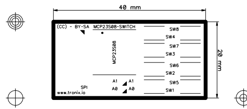
MCP23S08-SWITCH - (09/2017) - SCALE: 100%
