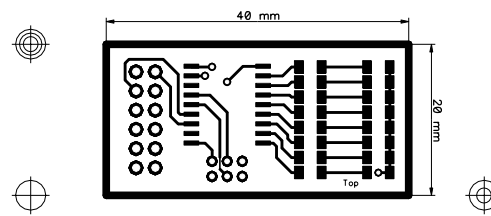
MCP23S08-LED - (12/2017) - SCALE: 100%
