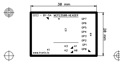
MCP23S08-HEADER - (12/2017) - SCALE: 100%
