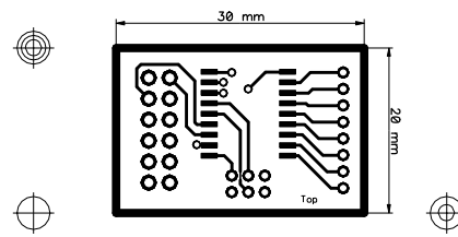
MCP23S08-HEADER - (12/2017) - SCALE: 100%
