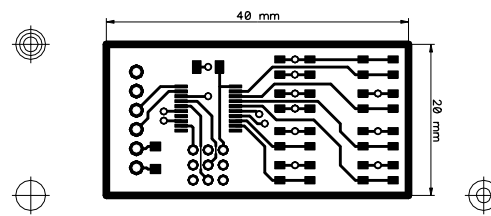
MCP23008-SWITCH - (12/2017) - SCALE: 100%
