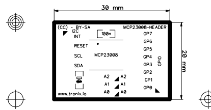
MCP23008-HEADER - (12/2017) - SCALE: 100%
