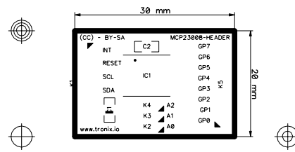
MCP23008-HEADER - (12/2017) - SCALE: 100%
