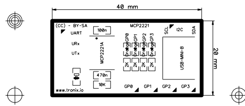
MCP2221 - (02/2018) - SCALE: 100%
