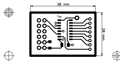
MC74HC595-HEADER - (01/2018) - SCALE: 100%
