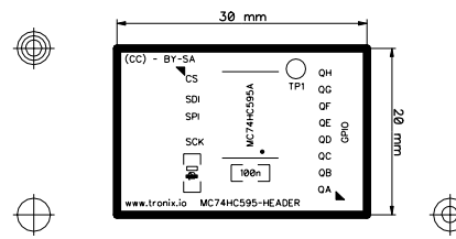
MC74HC595-HEADER - (01/2018) - SCALE: 100%
